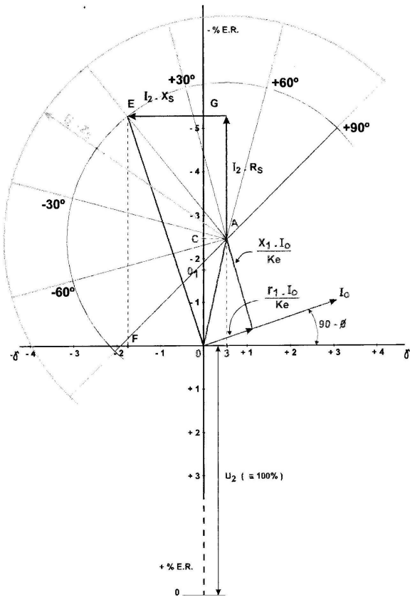
Fig. 7 Mollinger & Gewecke Diagram
