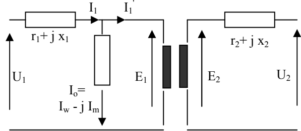
Fig. 4. T-Equivalent Transformer Model
